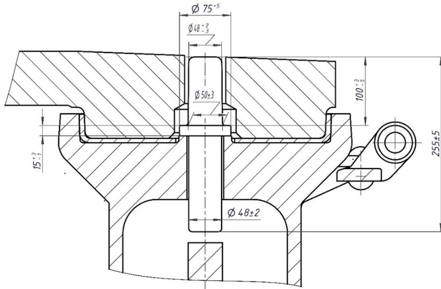
Рисунок А.1 – Шкворень
