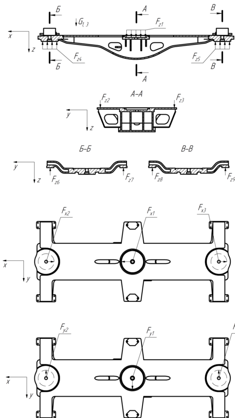
Рисунок В.1 – Схема сил, действующих на соединительную балку четырехосной тележки
