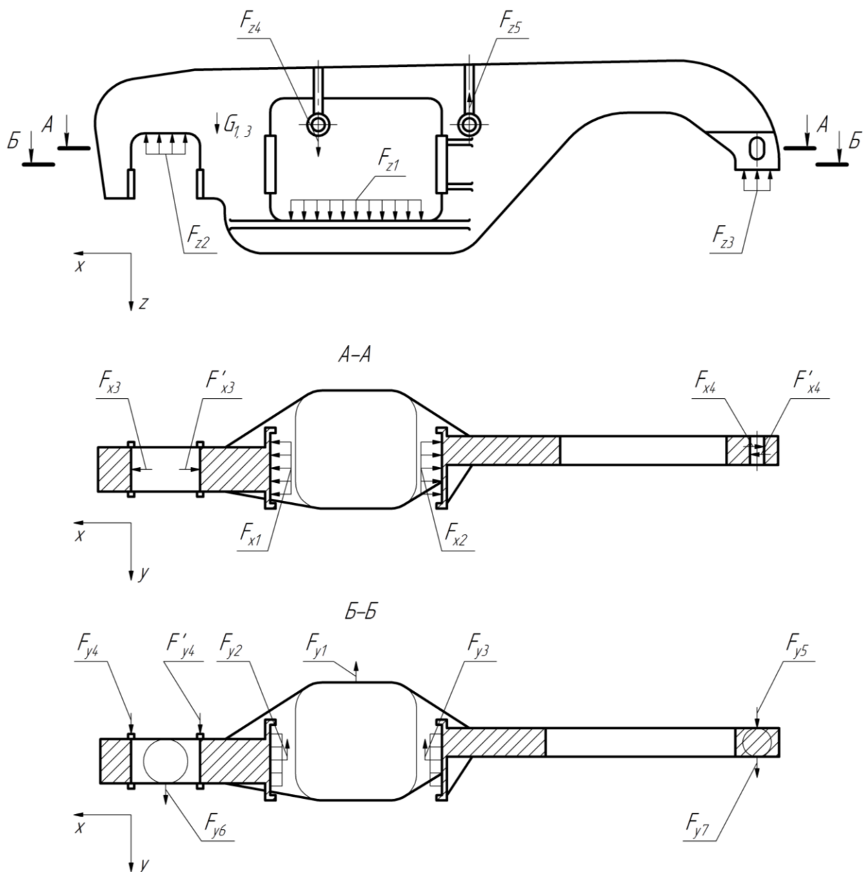
Рисунок Б.1 – Схема сил, действующих на боковую раму трехосной тележки
