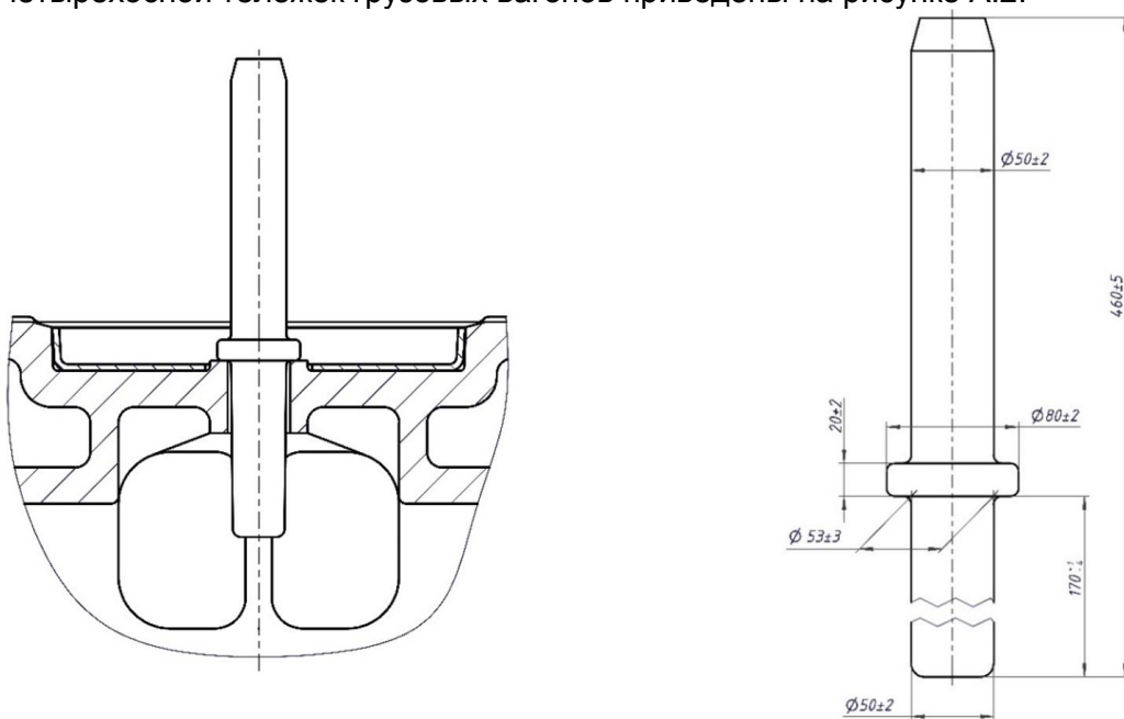
Рисунок А.2 – Шкворень
